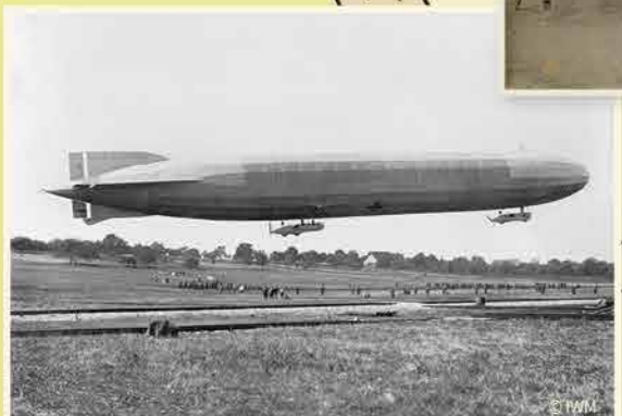
Zeppelin met twee gondels. 1915
